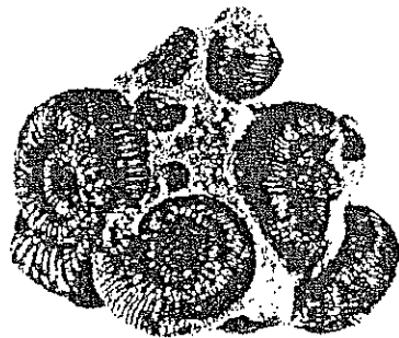
Stephanoceras humphreianum aus dem Dogger (Mitte Bojocum) von Garzen bei Alföld, GröÙe: 19 x 14 cm
