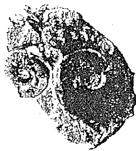
Dufrenoyia romani aus dem Dogger (Mitte Bojocum) von Garzen bei Alföld, GröÙe: 12 x 8 cm
